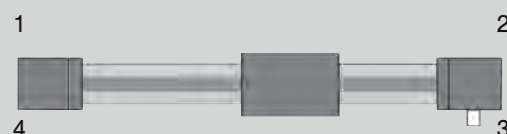
Arbre pour raccordement d'encodeur en 3 Option: G3 (ZK-255-3 \varnothing 25, ZK-405-3 \varnothing 40)
