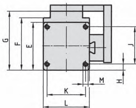
Vue X
